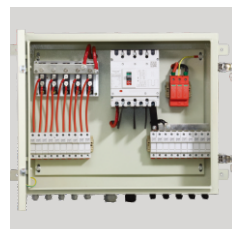
NSPV-10 MCCB+ Rectifier module/250
